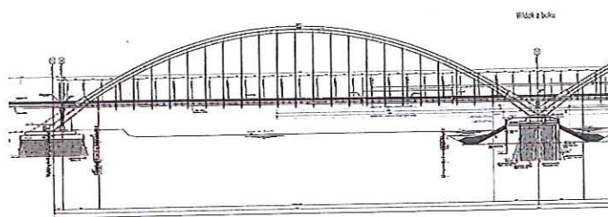
Rys. 2. Widok z boku przęsła północnego Źródło: Miejski Zarząd Dróg w Toruniu
